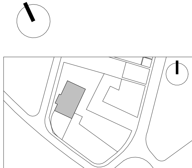
РАЗПРЕДЕЛЕНИЕ ЖИЛИЩНА ЧАСТ 5 ЕТАЖ (КОТА +13.00)
